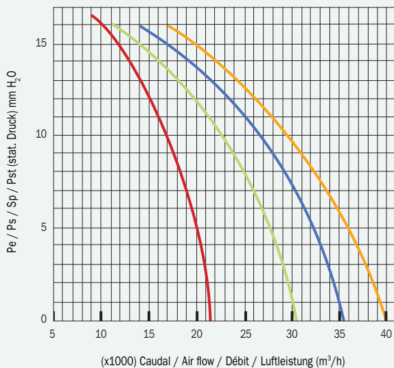
AXITUB EEX 900 RPM Ø 800
