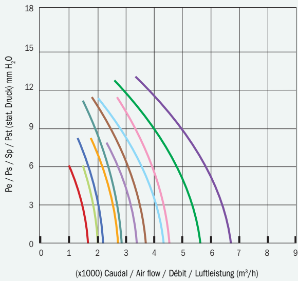
AXITEJ / AXITEJ BS 1400 RPM Ø 315-450
